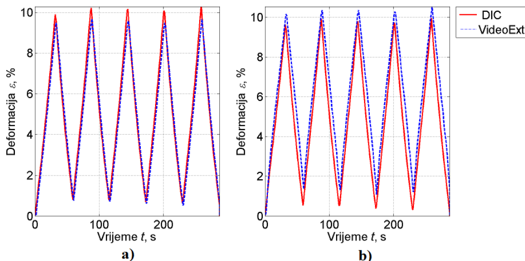
Slika 43. Usporedni prikaz promjene deformacije \epsilon u vremenu t za Prekondicioniranje 1 uzorka AORTA 1 u a) aksijalnom (A) i b) transverzalnom (T) smjeru za DIC i videoekstenzometar
