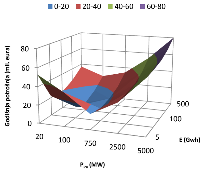
Grafikon 1 : Ukupni godišnji trošak u ovisnosti o instaliranom PV-u i spremniku el. energije 1. scenarija
