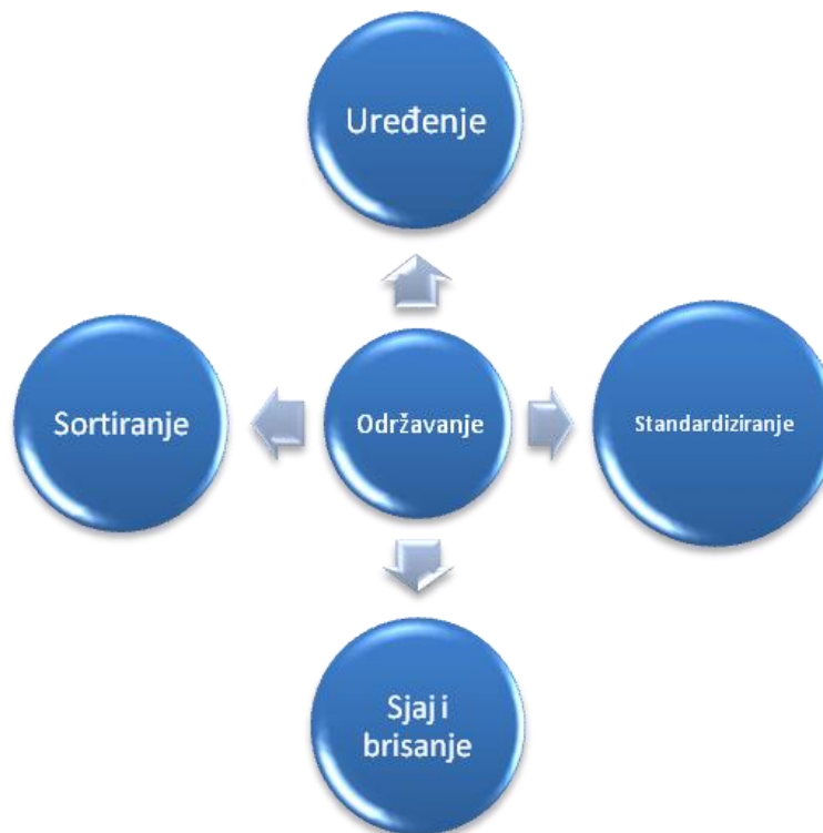
Slika 9. 5S metoda.
