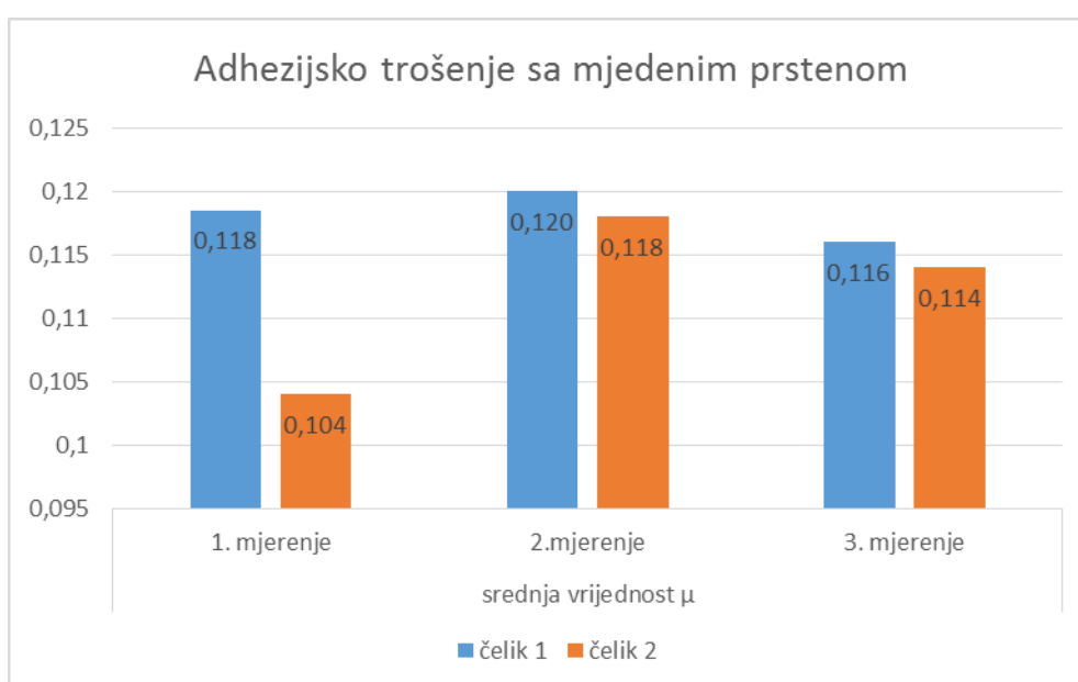
Slika 30. Srednje vrijednosti faktora trenja za čelike 1 i 2
