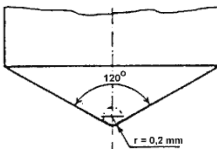
Slika 16. Rockwell C indentor [12]
