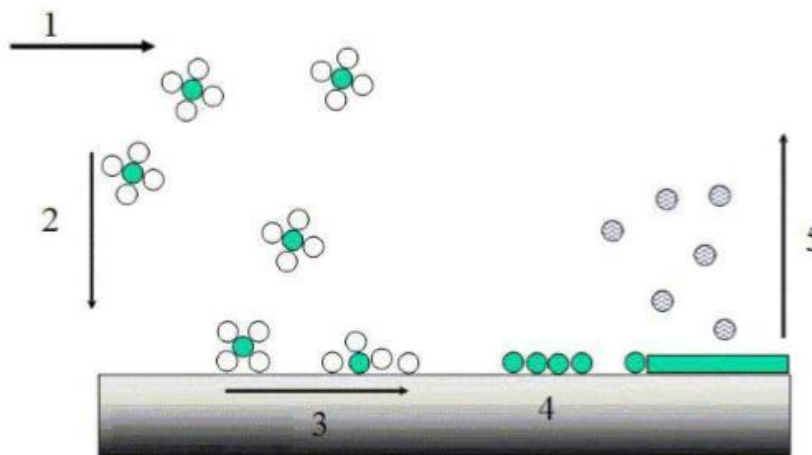
Slika 12. Faze stvaranja sloja u CVD postupaku prevlačenja [7]
