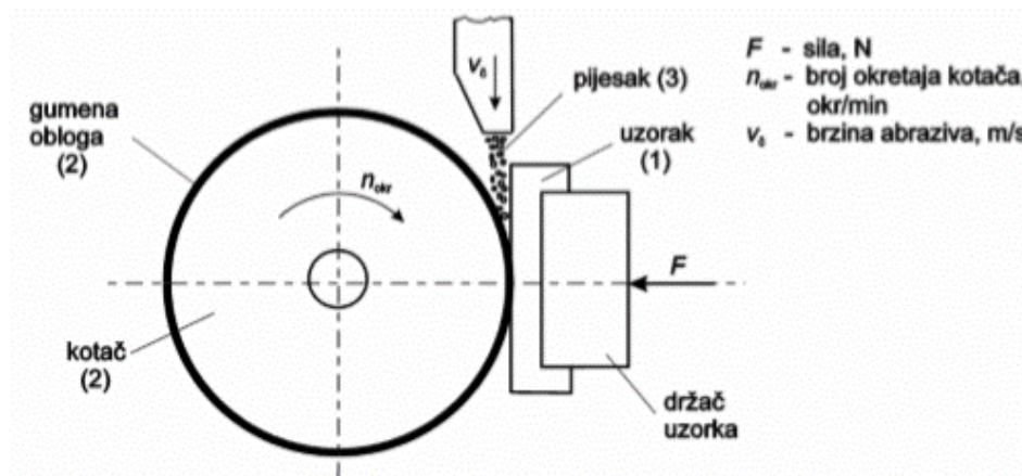
Slika 23. Skica uređaja „suhi pijesak/gumeni kotač“ [15]
