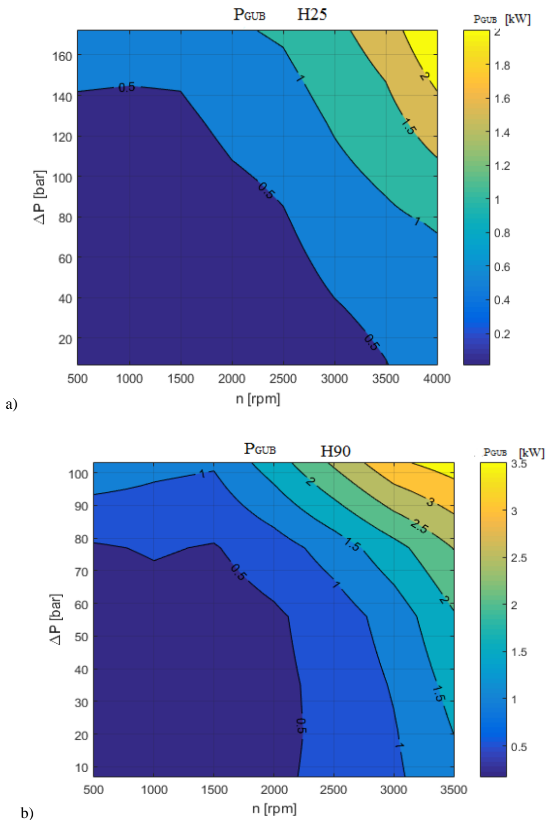
Slika 8.4 Karakteristike gubitaka za pumpe: a) H25, b) H90
