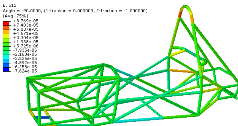
Slika 34. Posmične deformacija
