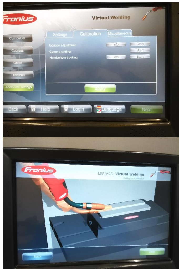
Slika 4.4. Kalibracija
