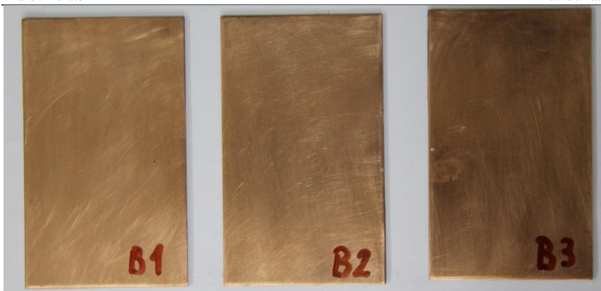
Slika 38. Rezultati ispitivanja uzoraka od bakra PE folijom debljine 120 \mu\text{m} u vlažnoj komori
