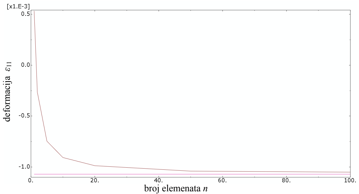
Slika 29. Konvergencija deformacija
