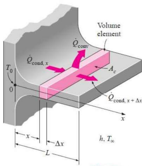
Slika 9. Obujam elementa [5]
