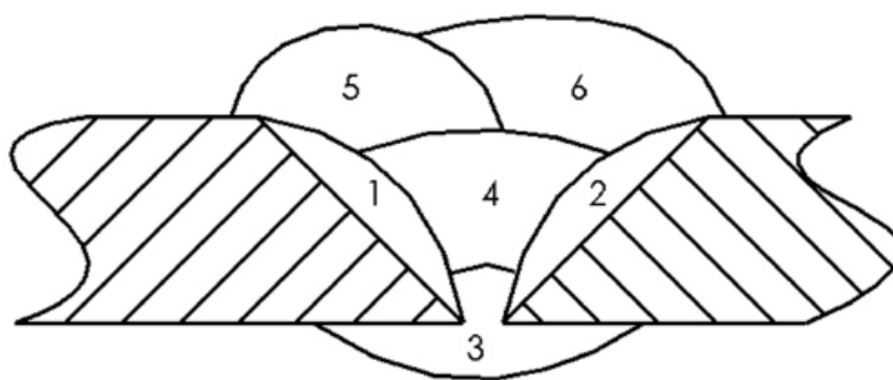
Slika 21. Redoslijed zavarivanja uzoraka U1, U3 i U4 [3]
