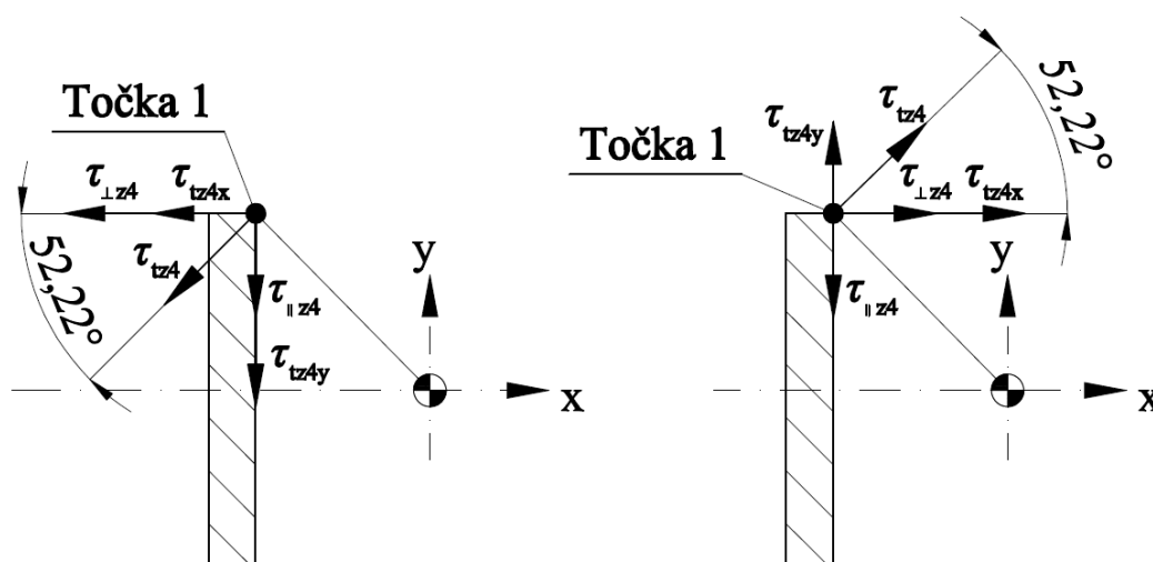
Slika 47: Smična naprezanja u točki 1 zavara 4, kada se uže nalazi bliže točke 1 (lijevo) i kada se uže nalazi dalje od točke 1 (desno)
