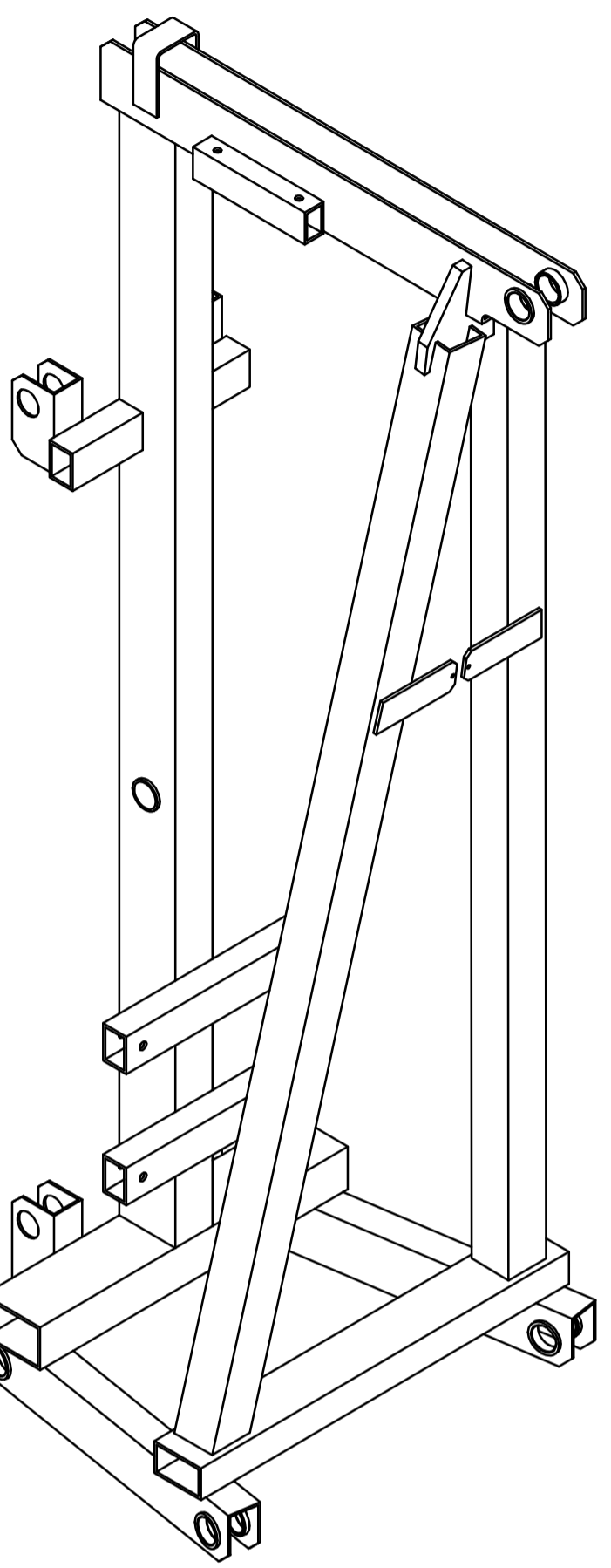
Izometrija (M1:10)
