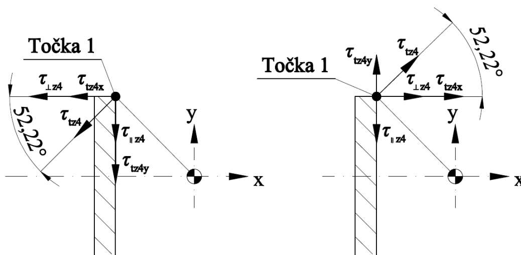
Slika 47: Smična naprezanja u točki 1 zavara 4, kada se uža nalazi bliže točke 1 (lijevo) i kada se uža nalazi dalje od točke 1 (desno)
