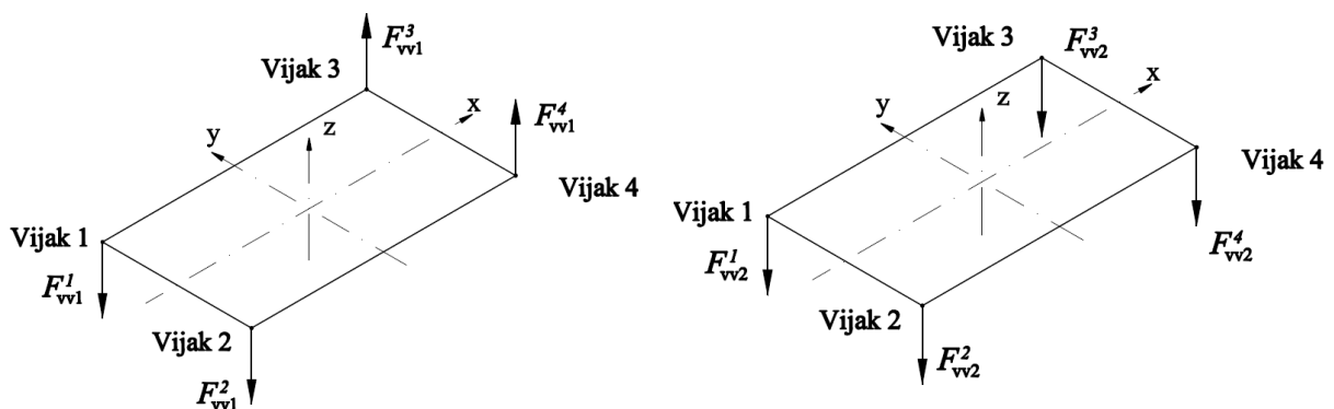
Slika 37: Sile u vijcima
