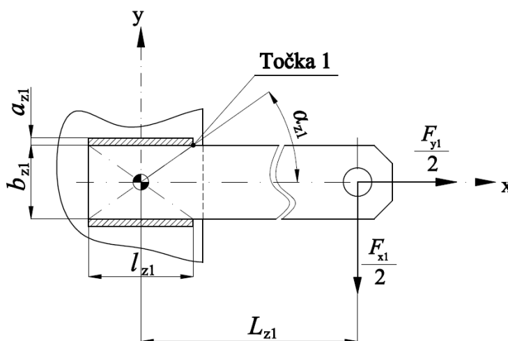
Slika 26: Geometrija zavara 1
