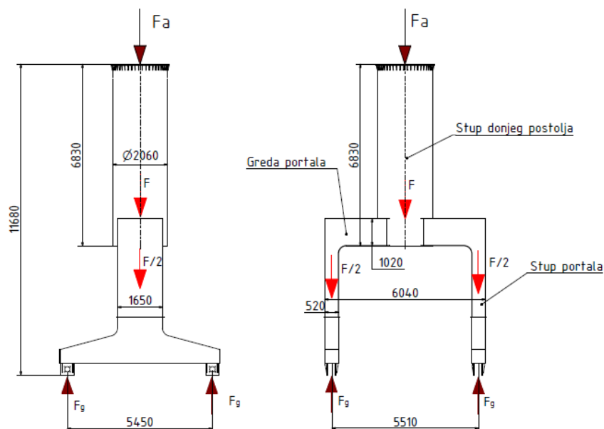
Slika 5.13. Shema sila na portal granika
