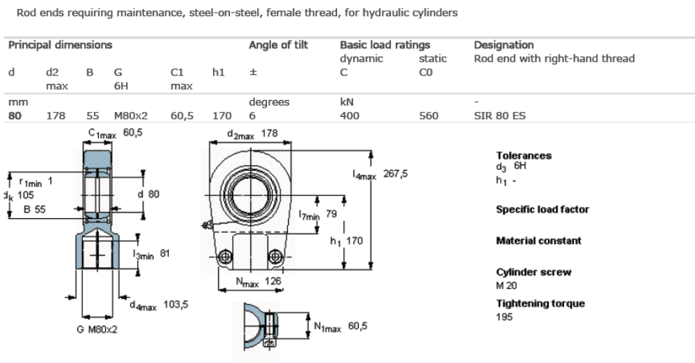
Slika 9.4. Kraj zubne letve SIR 80 ES, SKF
