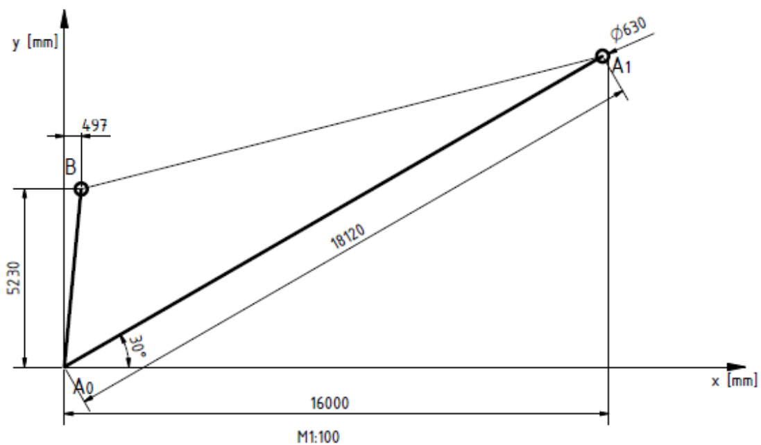
Slika 5.1. Shematski prikaz dohvatnika u mjerilu M 1:100
