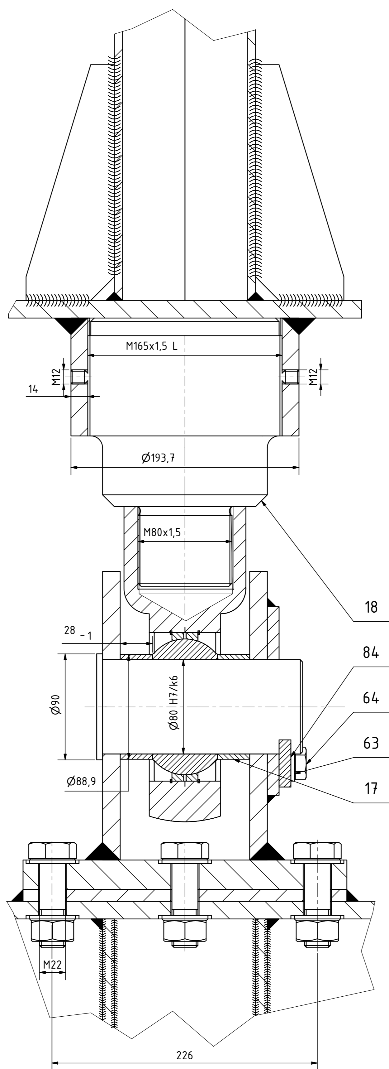
JA-JA ( 1 : 5 )
