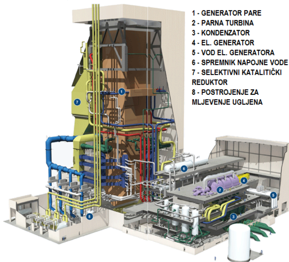
Slika 33. Prikaz nadkrićnog postorjenja sa svim dijelovima
