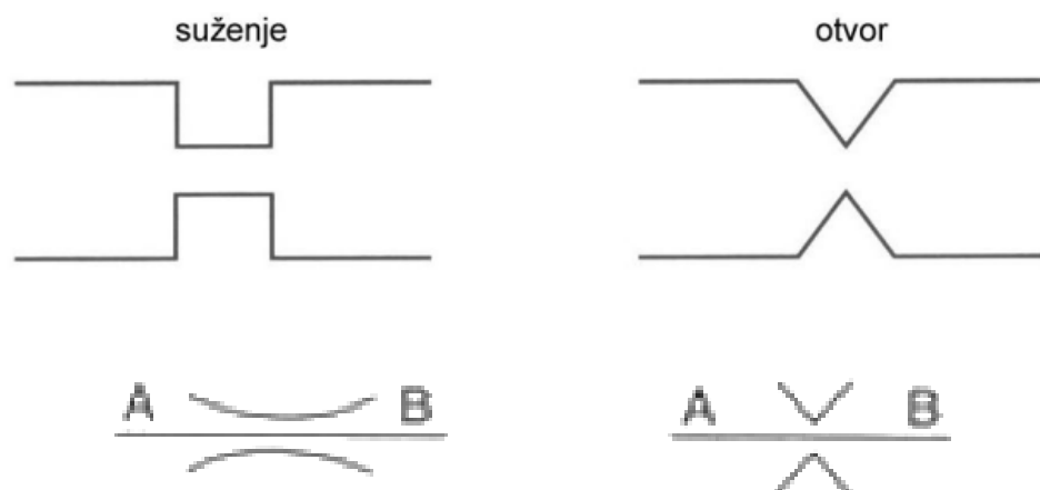
Slika 25. Prigušnica (lijevo) i blenda (desno)
