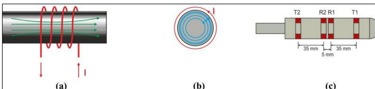
Slika 14. (a) Eksterna zavojnica za ispitivanje žice, (b) Smjer vrtložnih struja, (c) sonda za interno ispitivanje cijevi izmjenjivača toplote
