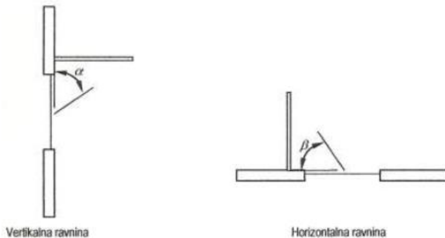
Slika 4.3. Prozorsko zasjenjenje: a) vertikalna ravnina, b) horizontalna ravnina [12]
