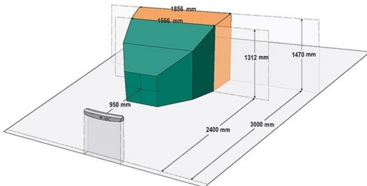
Slika 3.3: Polaris Spectra – mjerni volumen
