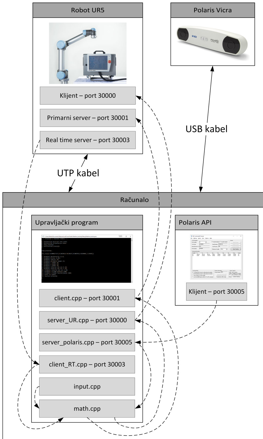
Slika 5.2: Shema sustava
