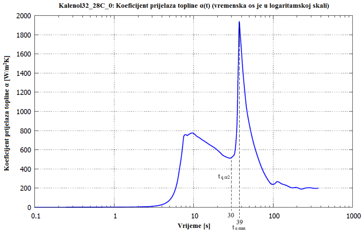
Slika 74. Koeffcijent prijelaza topline u ovisnosti o vremenu za gašenje u ulju Kalenol 32
