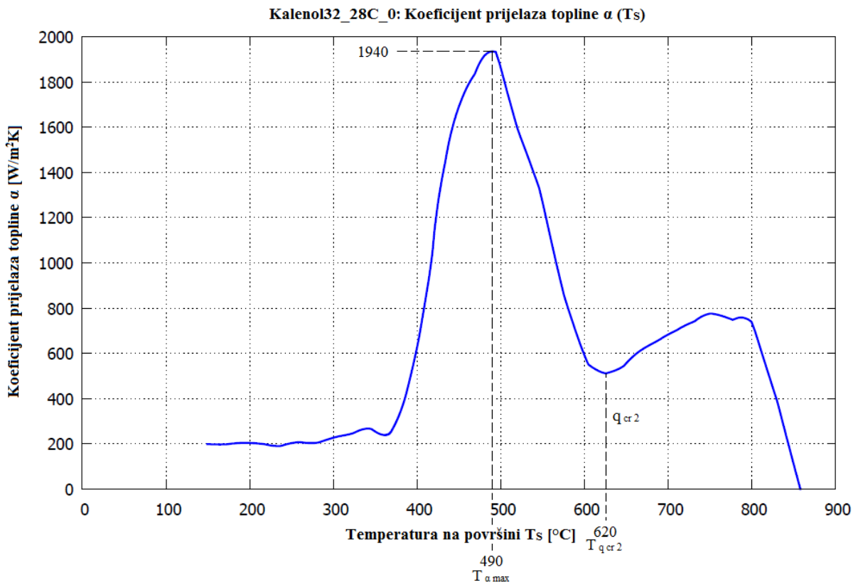
Slika 75. Koeffcijent prijelaza topline u ovisnosti o temperaturi na površini za gašenje u ulju Kalenol 32
