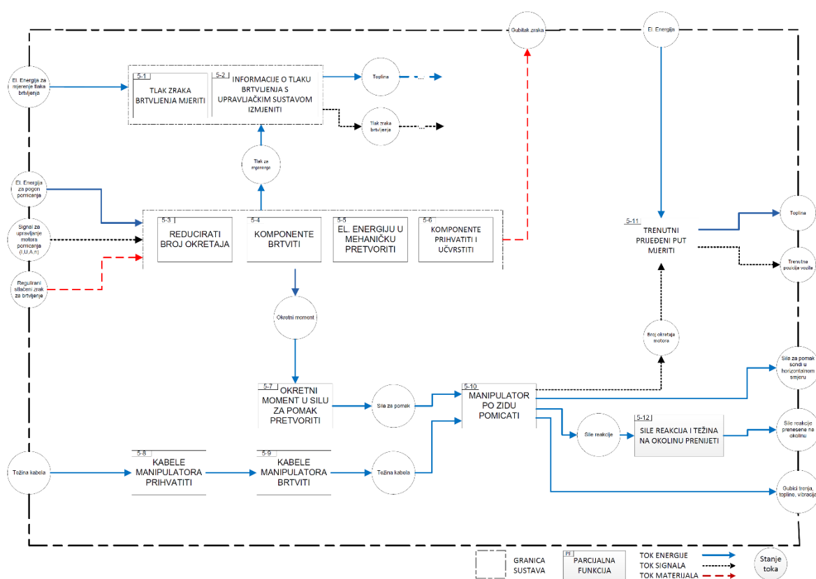
Slika 41. Funkcijska dekompozicija
