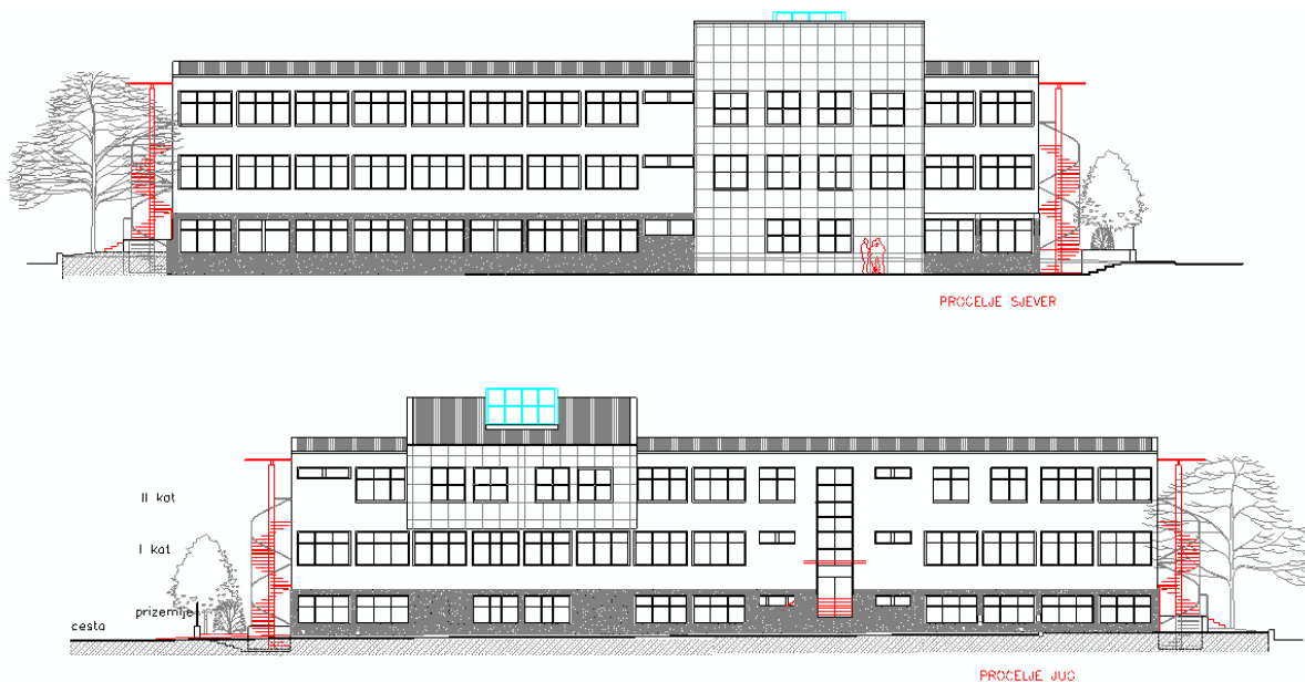
Slika 7. Sjeverno i južno pročelje poliklinike
