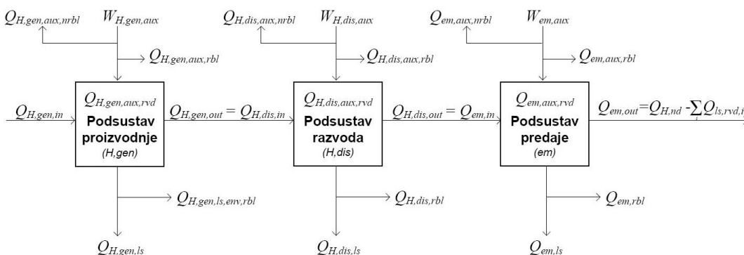
Slika 4. Podjela termotehničkog sustava grijanja i pripreme potrošne tople vode na podsustave s prikazom ulazno/izlaznih veličina [4]
