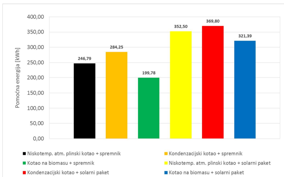
Dijagram 19. Rezultati ukupne pomoćne energije za razne podsustave proizvodnje - klimatsko područje Splita, Q_{H,nd}=10 \text{ kWh/m}^2
