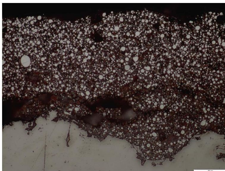
Slika 48. Mikrostruktura uzorka H, povećana 500 puta na svjetlosnom mikroskopu
