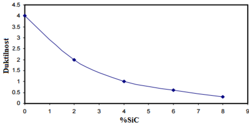
Dijagram 5: Utjecaj sadržaja SiC na duktilnost [16].
