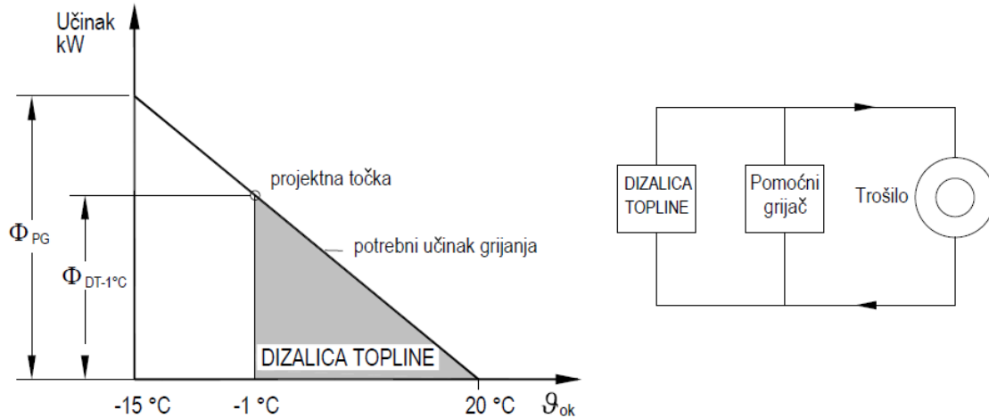
Slika 4. Bivalentno-alternativni način rada dizalice topline [3]
