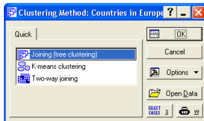
Slika 5. Odabir tipa klaster analize [4]
