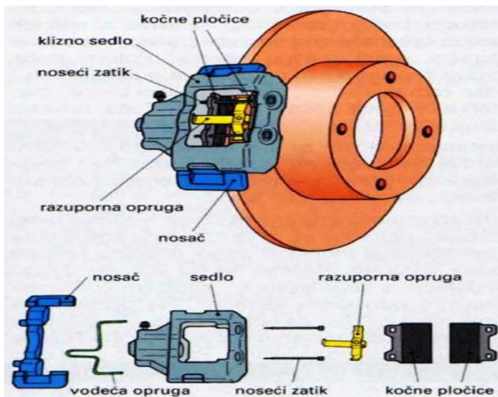
Slika 37. Disk kočnica s kliznim okvirom i vodećim zubom
