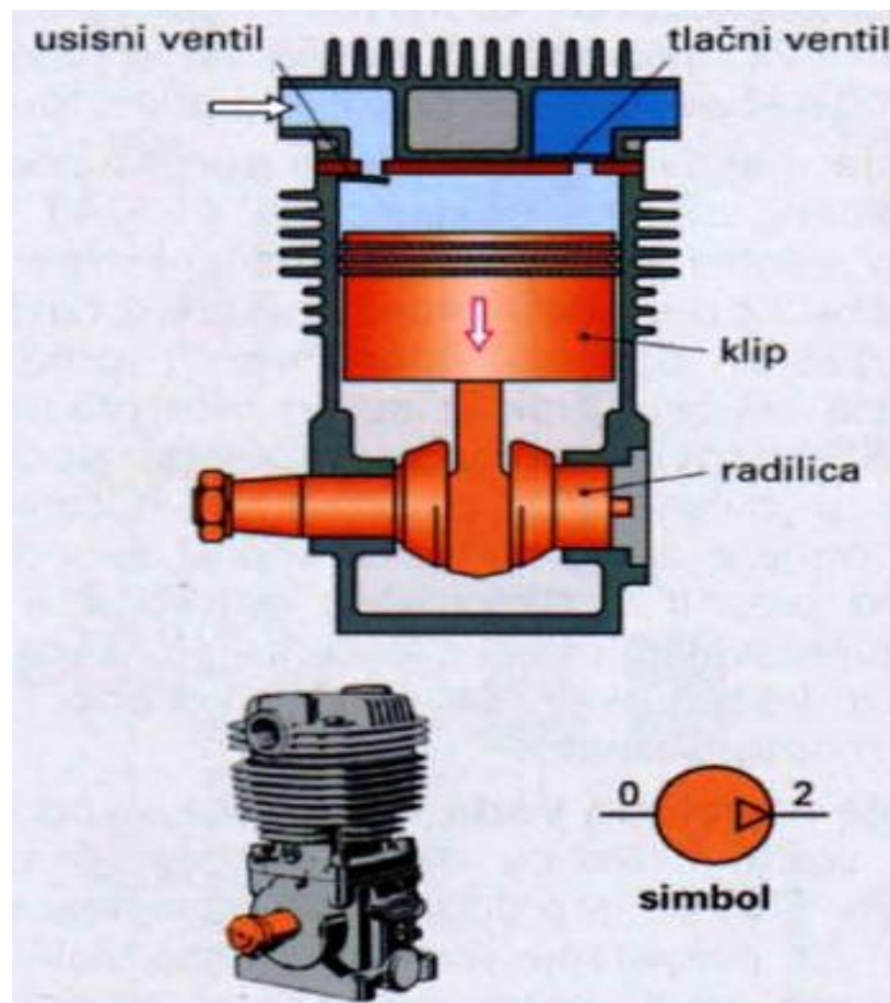
Slika 25. Kompresor
