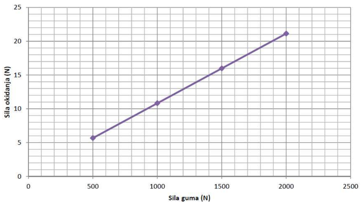
Slika 32. Ovisnost sile okidanja o sili guma
