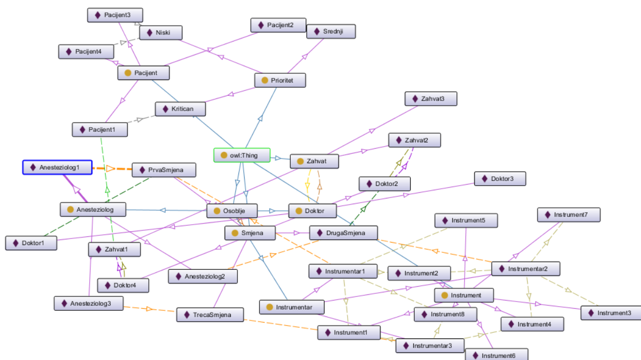
Slika 10. Onto Graph
