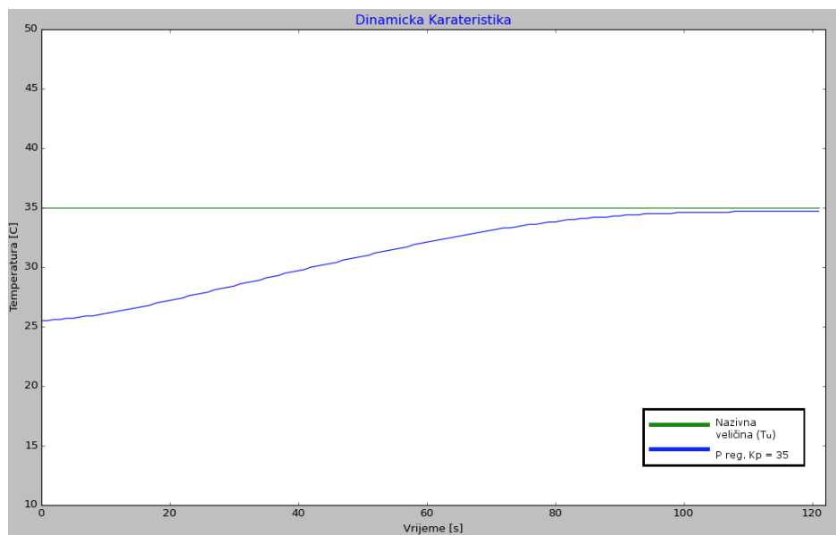
Slika 15. Odziv P regulatora
