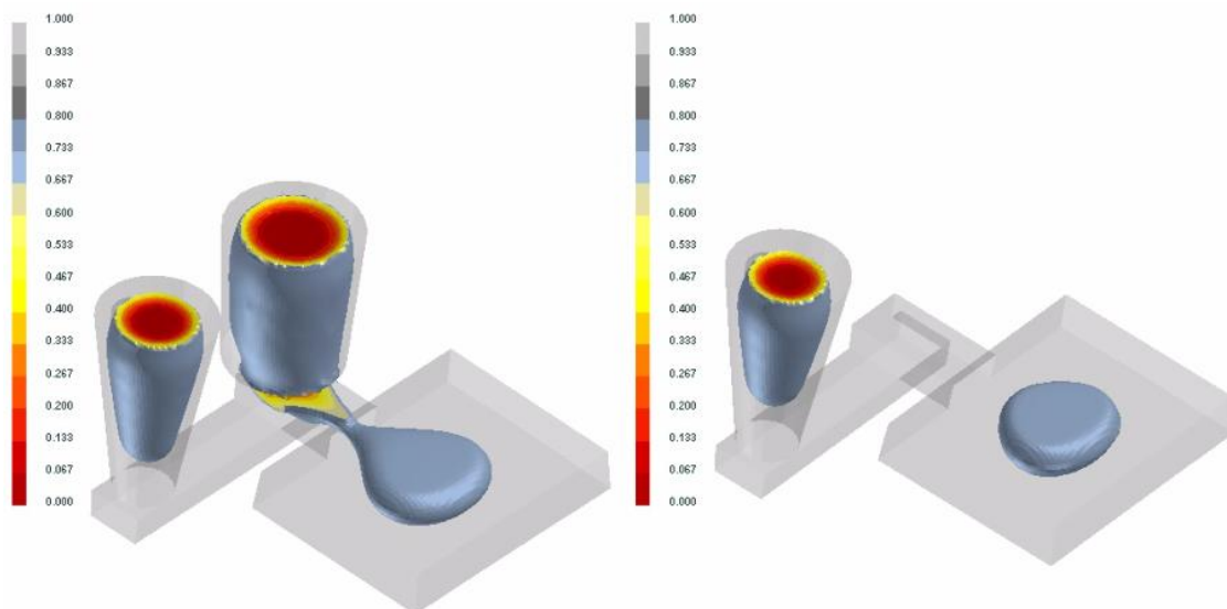
Slika 44: Završna mjesta skrućivanja u dvije različite varijante horizontalnog uljavnog sustava s i bez toplog pojila
