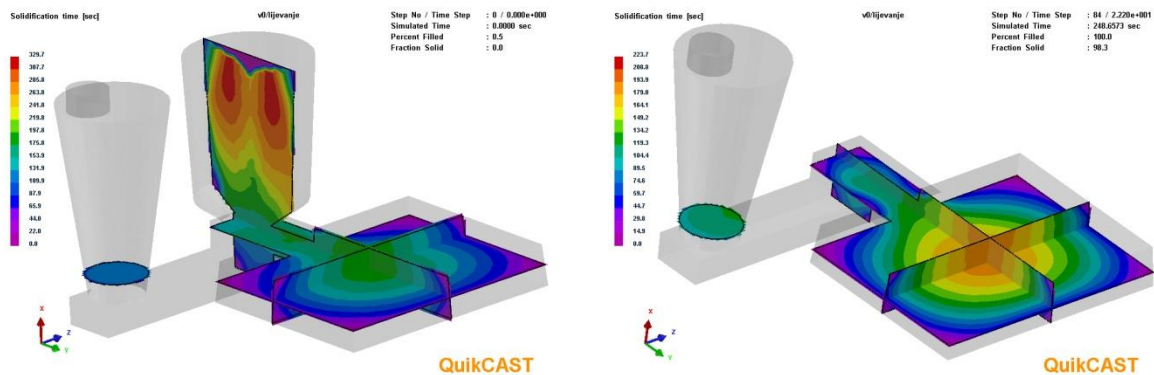
Slika 43: Vrijeme do solidusa u dvije različite varijante horizontalnog uljavnog sustava s jednim ušćem s toplim pojilom i bez njega
