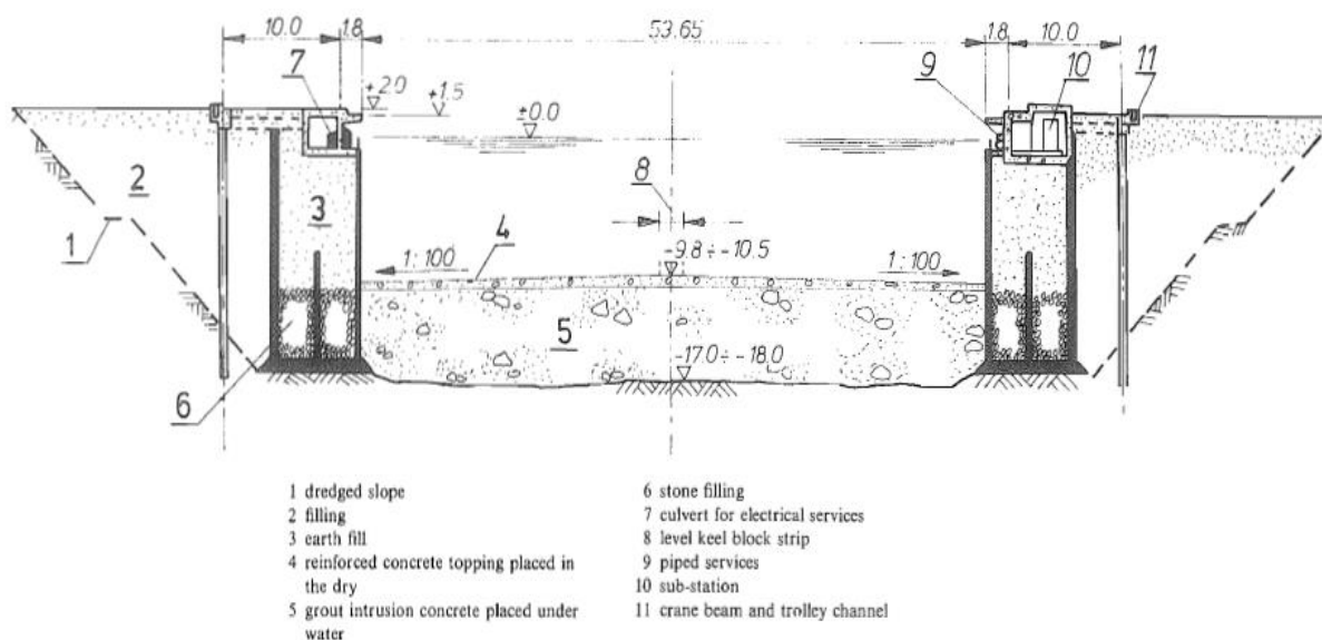
Slika 22. Presjek betonsko-masivnog suhog doka u Scaramangi [8]
