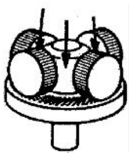
Slika 8. Ravna matrica [8]
