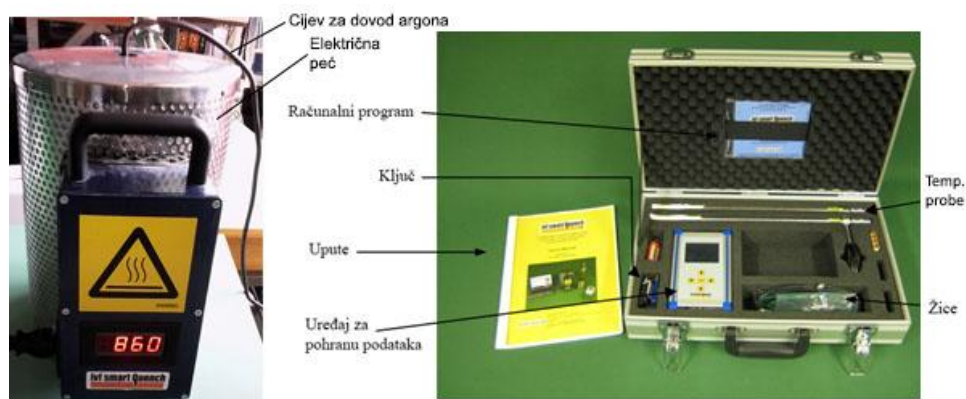
Slika 51. IVF Smart Quench oprema za ispitivanje krivulja hlađenja kapljevutih sredstava za gašenje [17]
