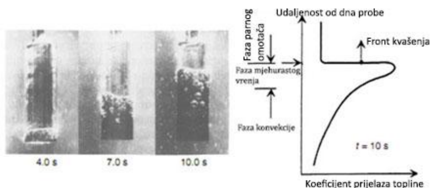
Slika 16. Napredovanje fronta kvašenja na čeličnom valjku [1]
