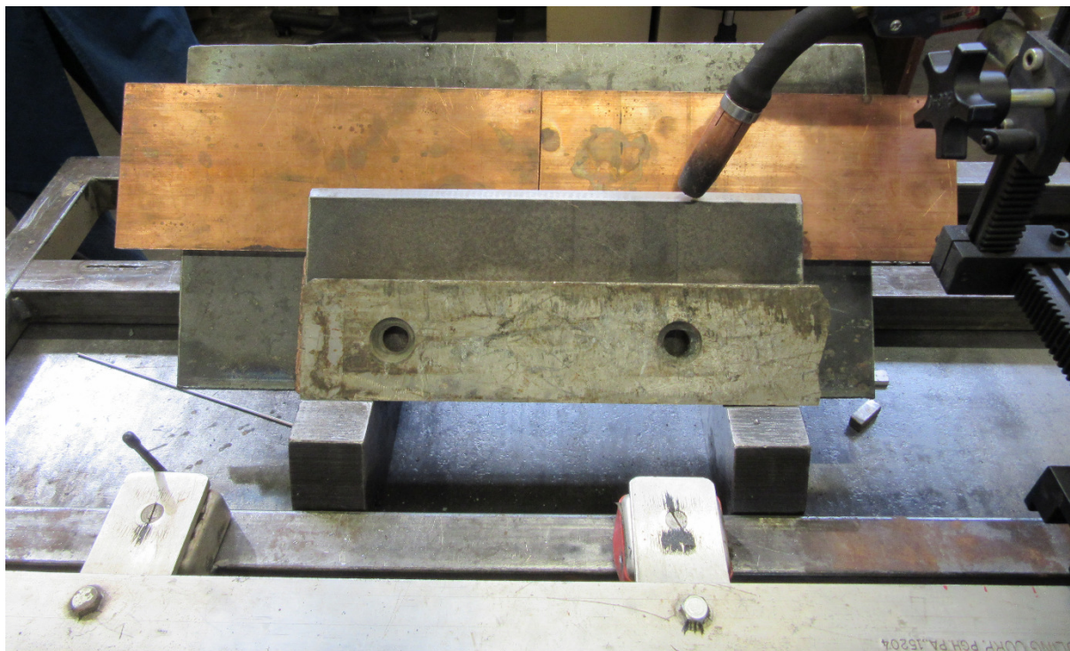
Slika 29 Konfiguracija zavarivanja međusloja
