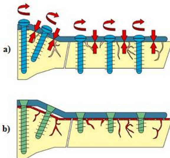
Slika 7. Očuvanje cirkulacije kod: a) konvencionalnih kompresijskih pločica i b) pločica na zaključavanje [18]
