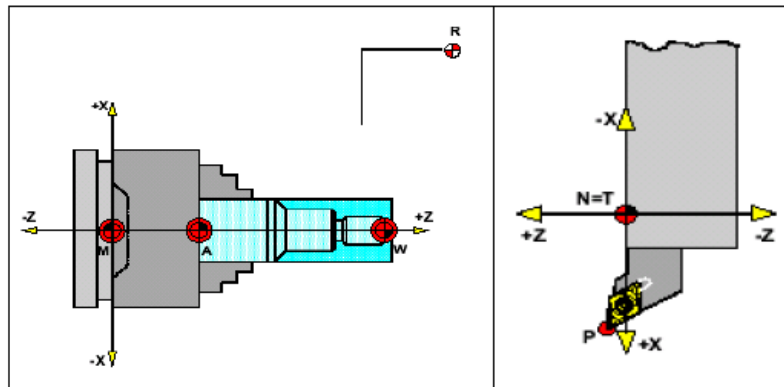
Slika 17. Prikaz nul točaka na NU tokarilici [1]
