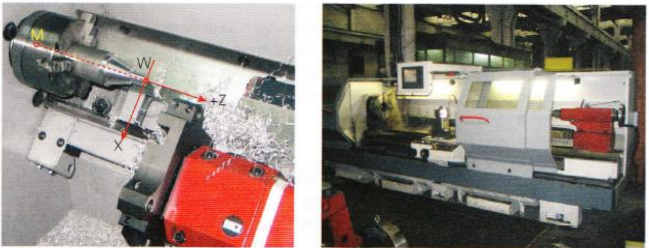
Slika 8. Horizontalna NU tokarilica [2]
