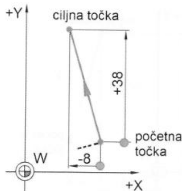
Slika 16. Inkrementalni koordinatni sustav [2]
