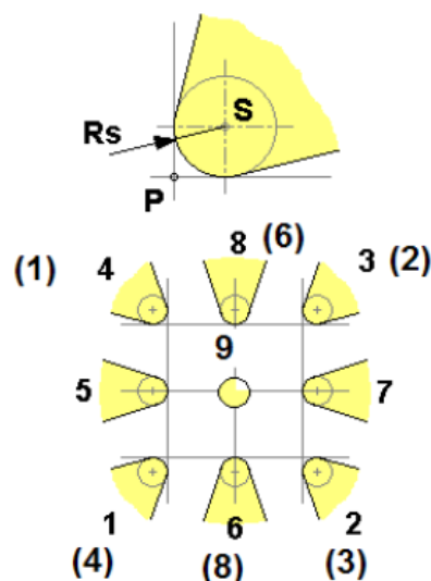
Slika 10. Položaj vrha oštrice alata [2]
