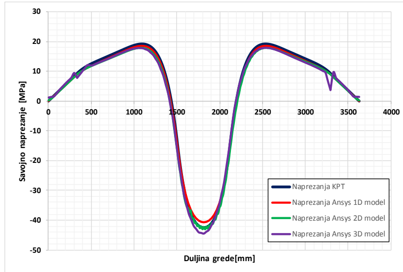
Slika 124. Usporedba savojnog napreznosti 1D, 2D, 3D i KPT modela
