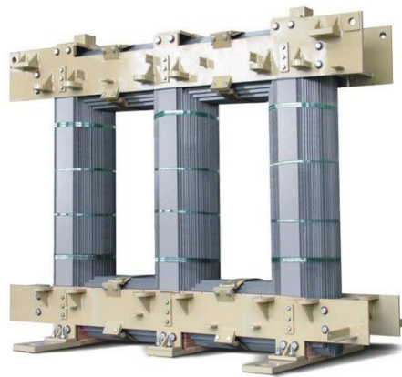
Slika 3. Stegnuta metalna jezgra transformatora od tankih limova [8]
