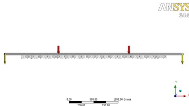
Slika 112. Rubni uvjeti i opterećenje grede na elastičnoj podlozi - Jezgra 2/0 s vijcima
