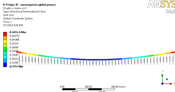
Slika 55. Raspodjela progiba
