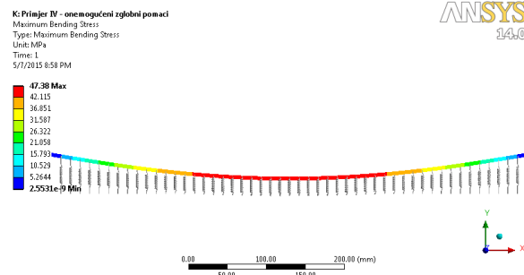
Slika 56. Raspodjela savojnog naprezanja
