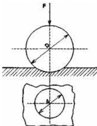
Slika 20. Skica kuglice i otiska kod Brinell-ove metode [31]
