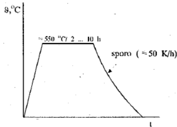
Slika 80. Dijagram postupka žarenja za redukciju zaostalih naprezanja[20]
