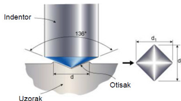
Slika 118. Prikaz indentora i otiska kod Vickersove metode[35]
