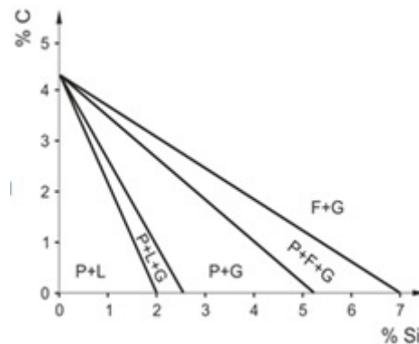
Slika 117. Klingensteinov strukturni dijagram[34]
