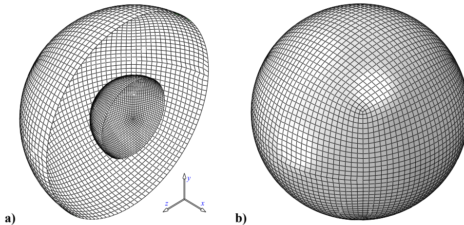
Slika 14.7. S4R deformirani oblik PM, p_i \approx 3,16 kPa, e_n \approx 1,56 : a) polovina modela, b) cijeli model
