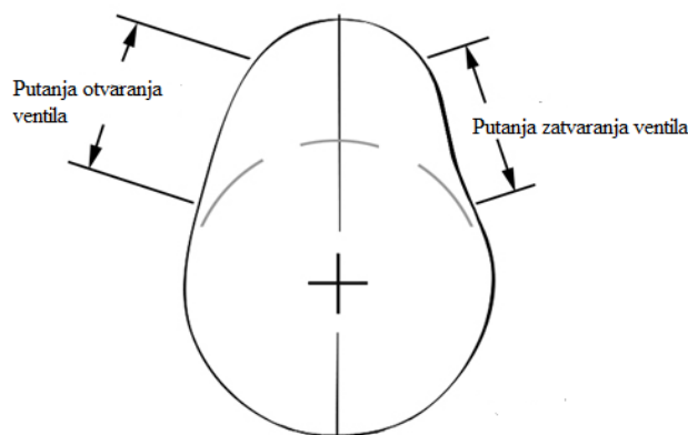
Slika 6. Primjer asimetrične konstrukcije brijega [7]
