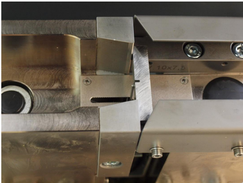
Slika 42. Centriranje uzorka
