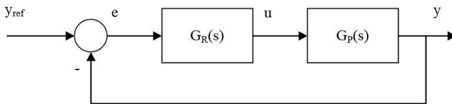
Slika 1. Upravljački krug
