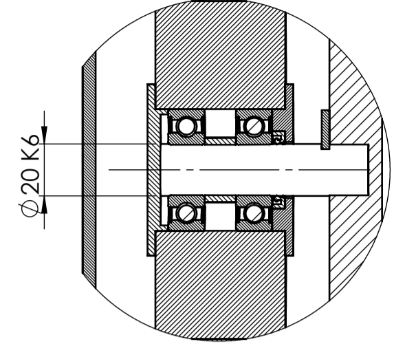
DETALJ B MJERILO 1:2
