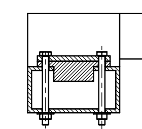
PRESJEK E-E M 1 : 5
