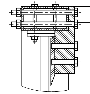
PRESJEK D-D M 1 : 5
