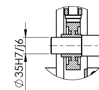
DETALJ H M 1 : 5
