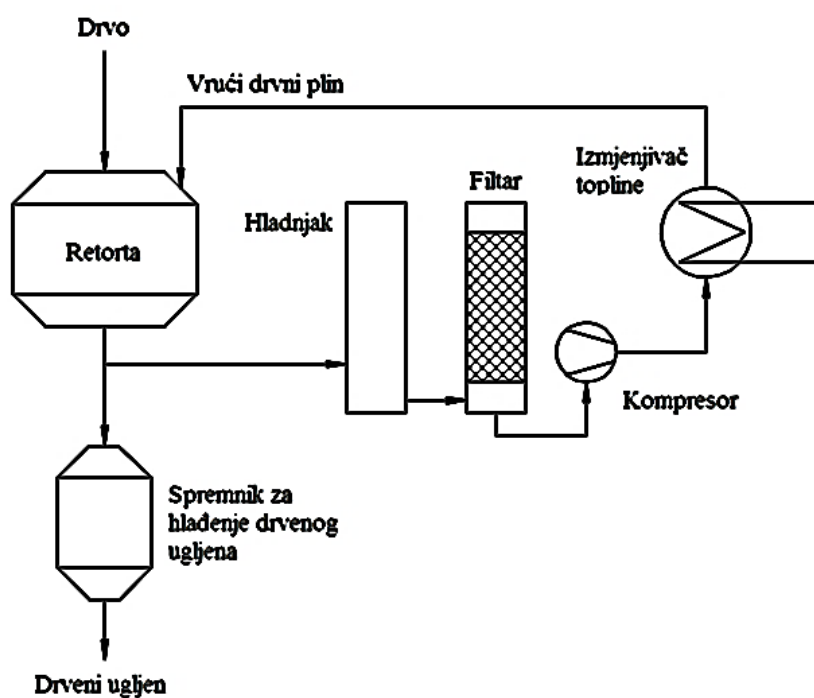
Slika 4: Degussa retorta
