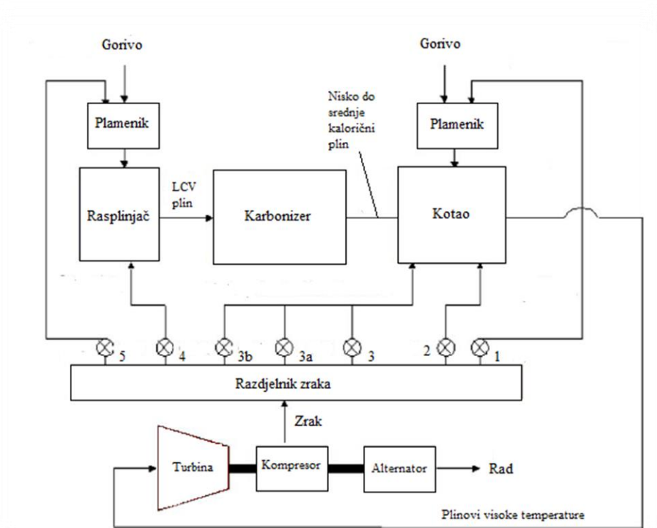
Slika 6: CHaP sustav [10]
