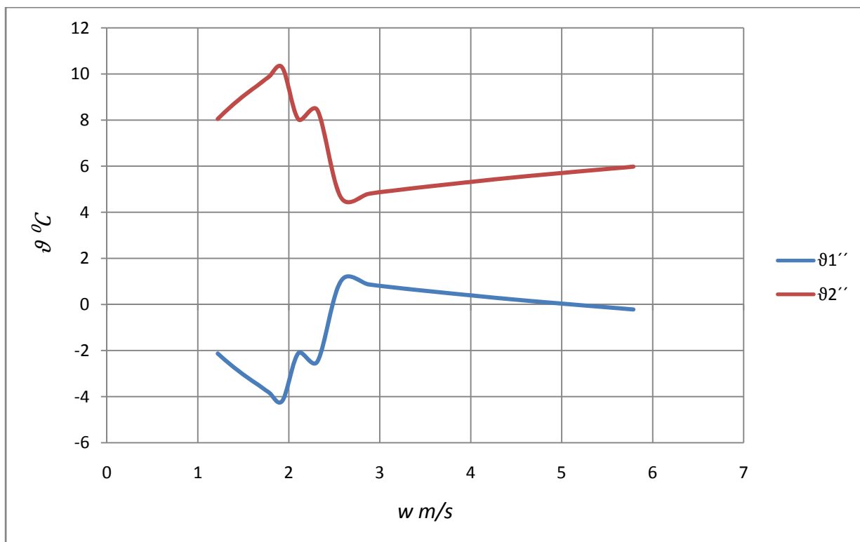
Slika 26. Ovisnost temperature ubacivanja svježeg zraka u prostoriju ( \theta_{1''} ) i temperature izbacivanja otpadnog zraka ( \theta_{2''} ) o brzini strujanja pri vanjskoj temperaturi \theta_{1'} = -15^\circ\text{C}
