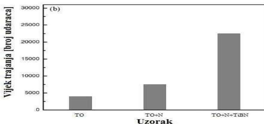
Slika 7. Vijek trajanja različito obradenih alata svrdla pri testu bušenja [8]
