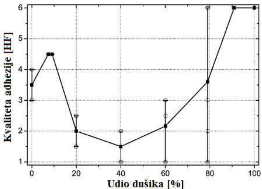
Slika 3. Adhezijske čvrstoća nitriranih uzoraka pri različitom omjeru plinova H_2/N_2 [11]
