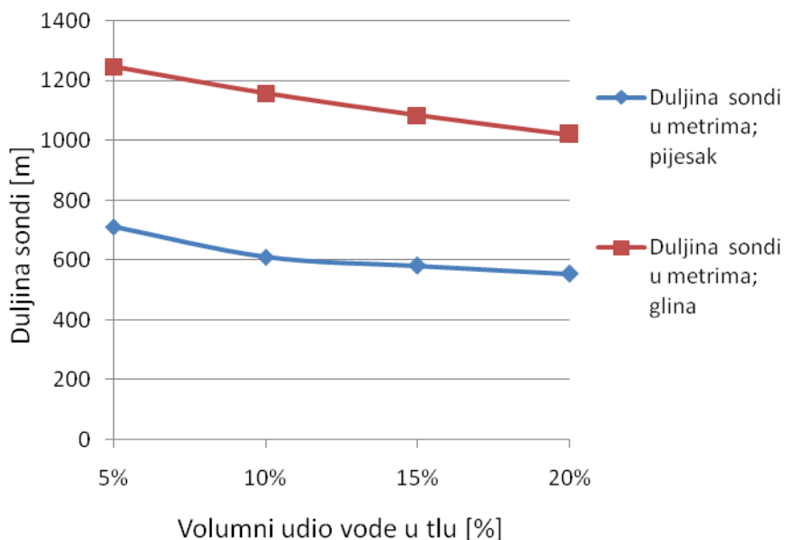
Slika 20. Utjecaj sadržaja vode u tlu na duljinu vertikalnih sonde
